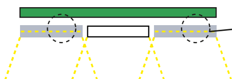
4,5 m Schiene für die gewählte Konfiguration von 3 Elementen: 3 Lichtlinie 1,5 m oder 2 Lichtlinie 1,5 m + 1 Blindsegment 1,5 m
