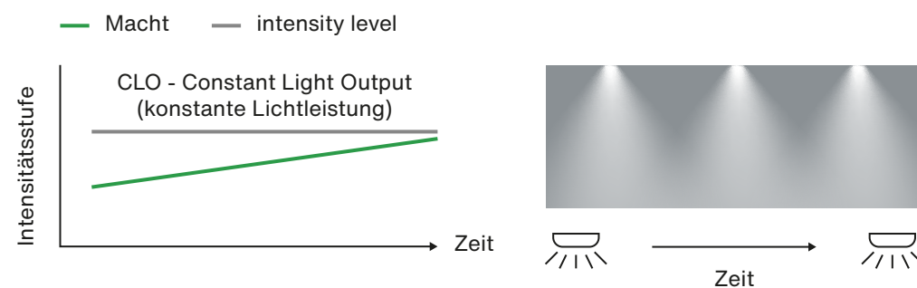
Lichtintensität im Zeitverlauf mit intelligenter Steuerung
