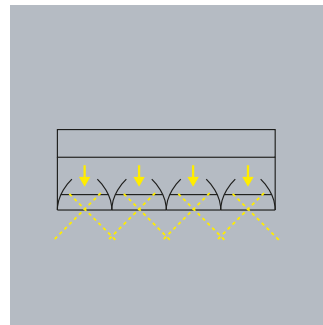
Auf spiegelnder Reflexion basierendes System
